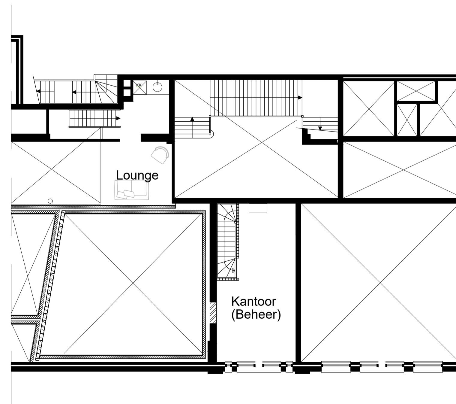
PLATTEGROND TUSSENVERDIEPING / ENTRESOLS
